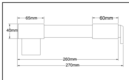
Dimensions
